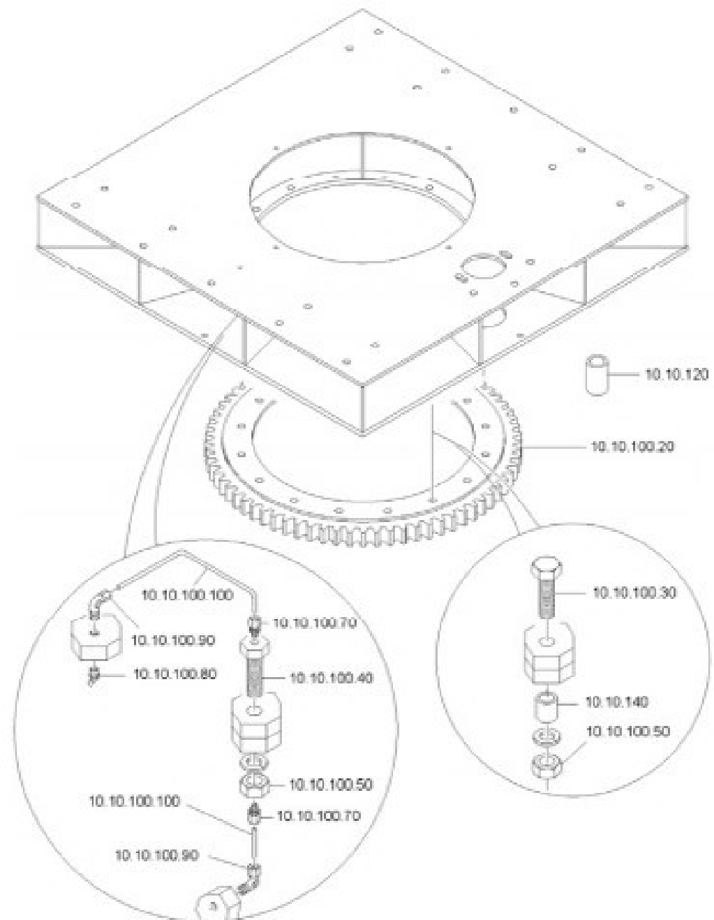
Abb. 03: Tragrahmen, kompl. Fig. 03: Supporting frame, compl. Fig. 03: Cadre porteur, compl. Fig. 03: Bastidor de soporte, compl.
